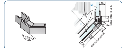
Art.-Nr. 8597KU7-L Fünfeckverbinder links-Türband rechts
