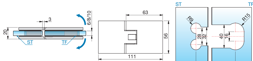
Glasbearbeitung für 8 mm Glas ohne Dichtprofil
