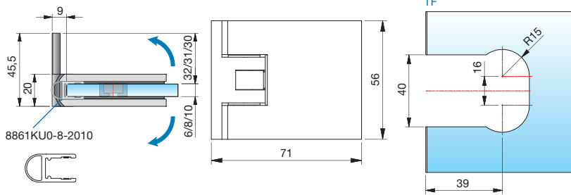
Glasbearbeitung für 8 mm Glas mit Dichtprofil 8861KUO-8-2010
