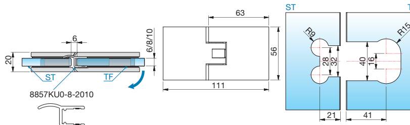
Glasbearbeitung für 8 mm Glas mit Dichtprofil 8857KUO-8-2010
