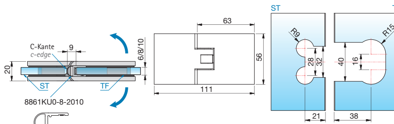
Glasbearbeitung für 8 mm Glas mit Dichtprofil 8861KUO-8-2010
