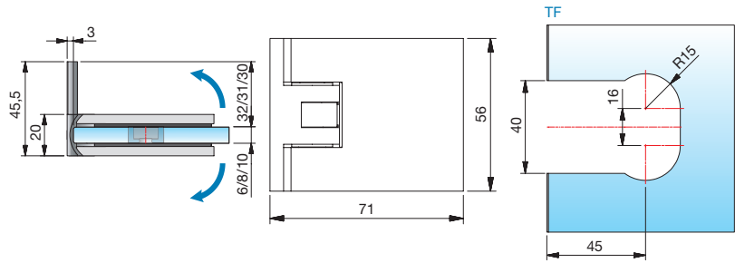
Glasbearbeitung für 8 mm Glas ohne Dichtprofil
