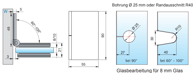
Glasbearbeitung für 8 mm Glas
