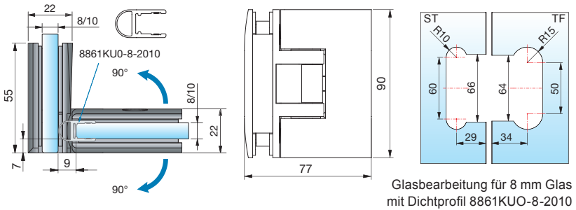
Glasbearbeitung für 8 mm Glas ohne Dichtprofil
