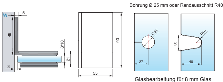
Glasbearbeitung für 8 mm Glas
