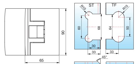
Glasbearbeitung für 8 mm Glas mit Dichtprofil 8861KU0-8-2010
