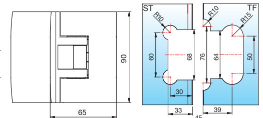
Glasbearbeitung für 8 mm Glas ohne Dichtprofil
