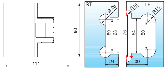
Glasbearbeitung für 8 mm Glas ohne Dichtprofil
