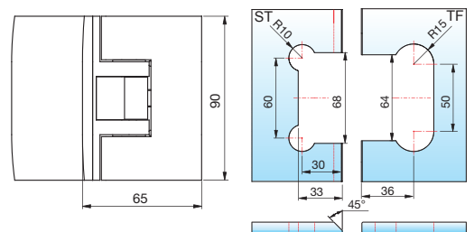
Glasbearbeitung für 8 mm Glas mit Dichtprofil 8860KU0-8-2010
