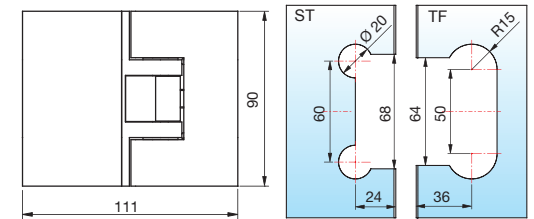
Glasbearbeitung für 8 mm Glas mit Dichtprofil 8857KU0-8-2010
