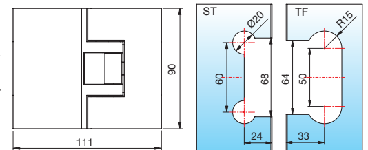
Glasbearbeitung für 8 mm Glas mit Dichtprofil 8861KU0-8-2010
