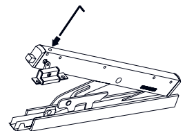
Schere mit Aushängesperre
