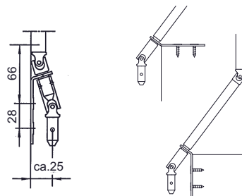
Kurbelstange abnehmbar
