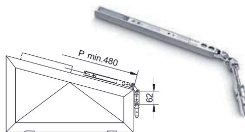
P = Länge des schrägen Schenkels
