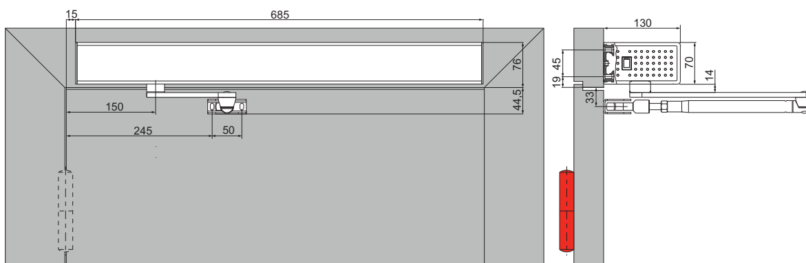
Achsverlängerung Standard
