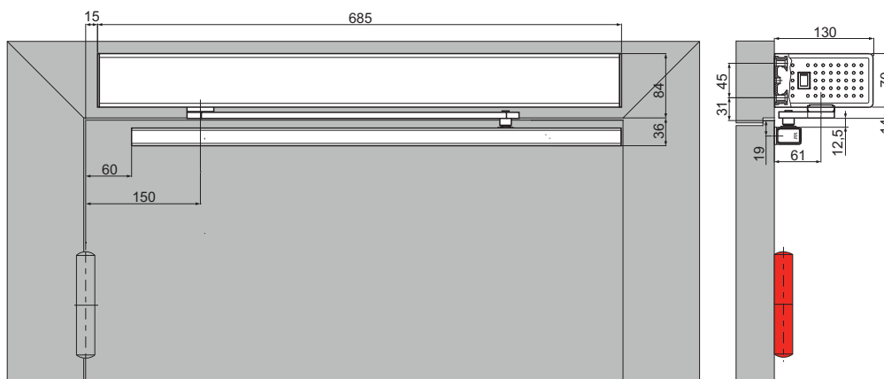
Achsverlängerung Standard
